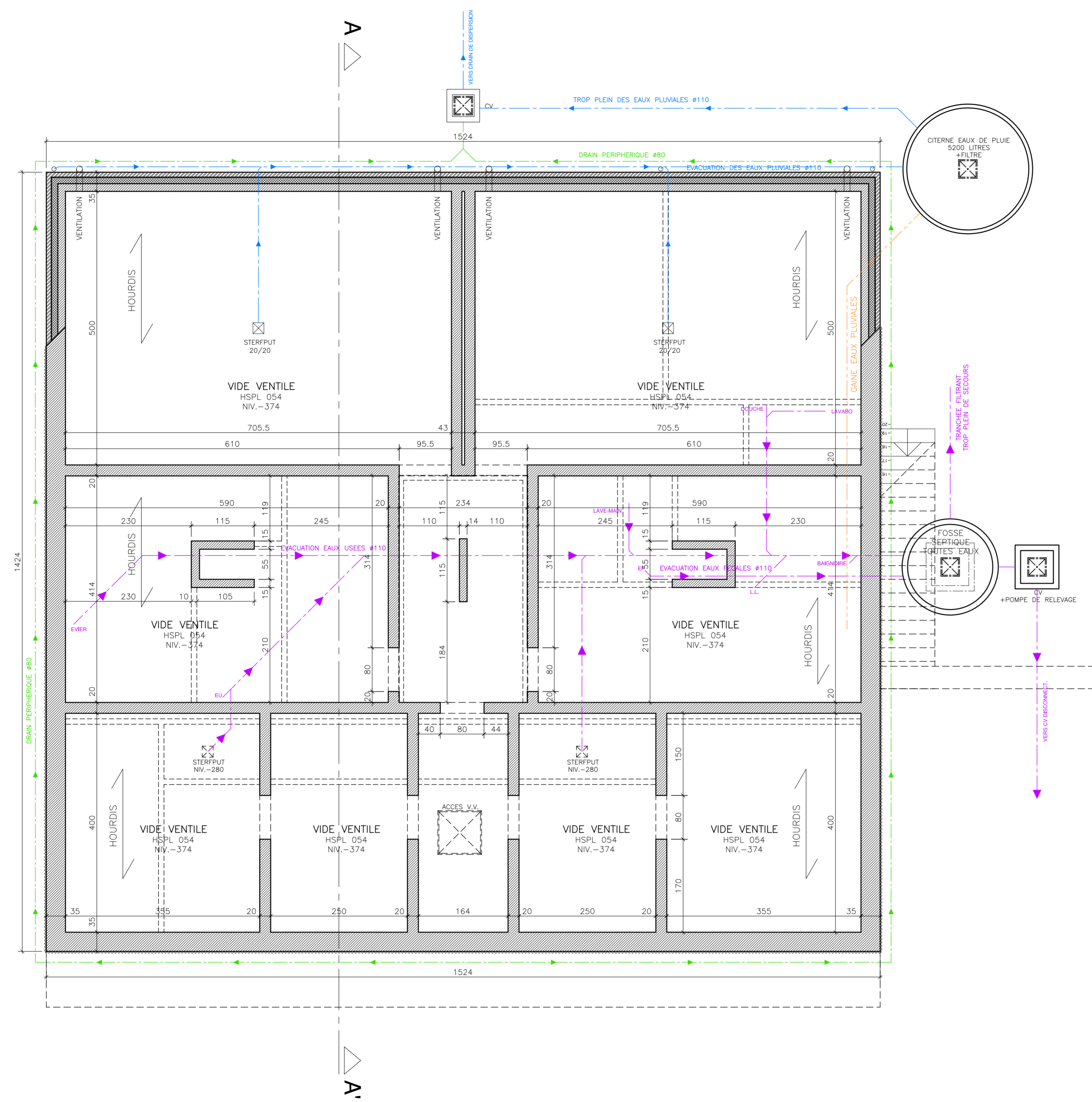
PLAN FONDATIONS
